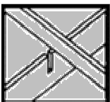
Pletinas desiguales encaste en pletina portante
